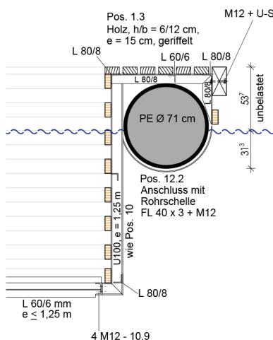
Längsschnitt Schwimmbeckenrand
